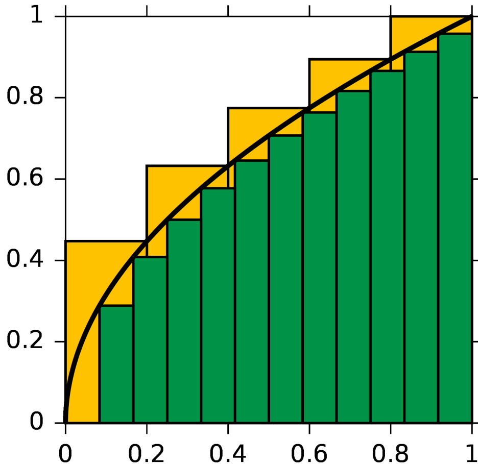
Figure 1. Riemann Sum.
